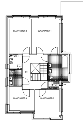
eerste verdieping
